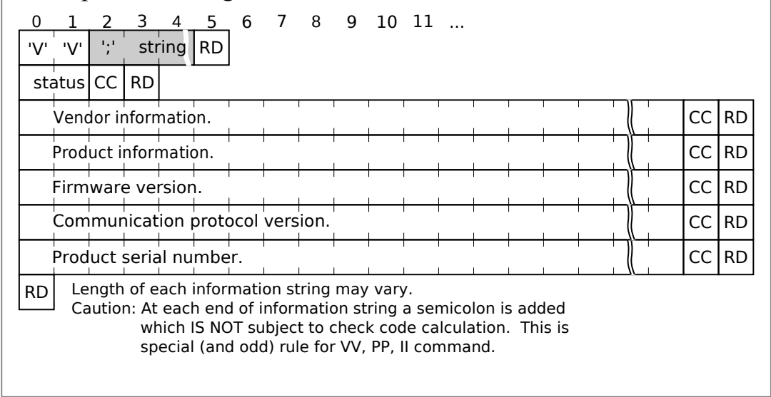
Figure 3.18 : VV Message Format
