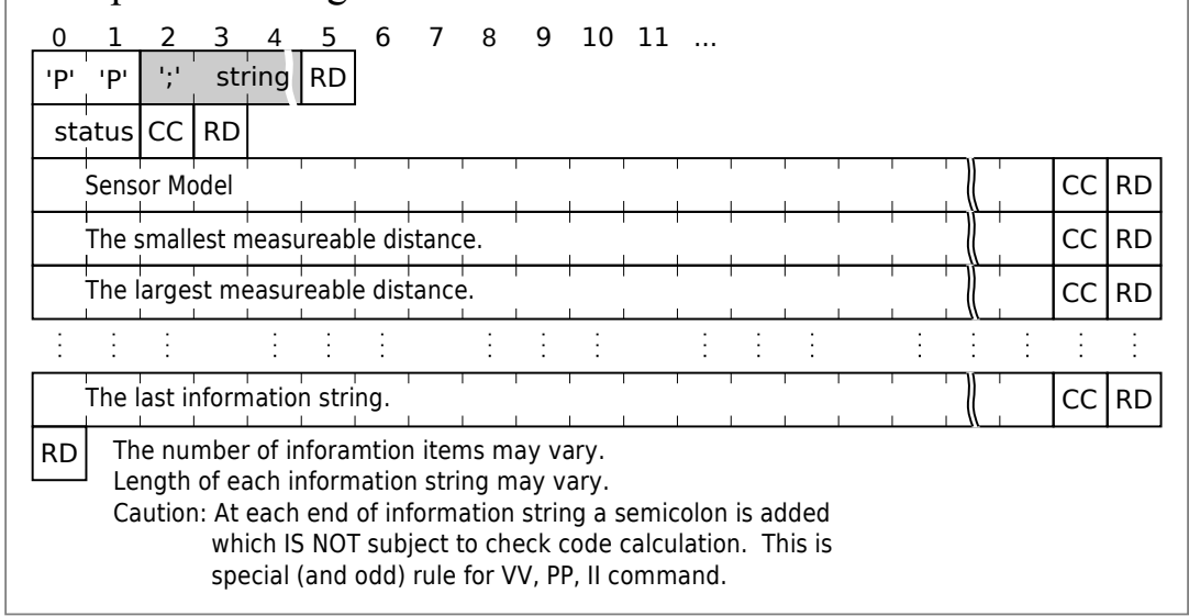
Figure 3.19 : PP Message Format
