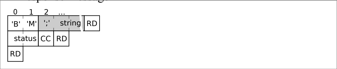
Figure 3.11 : BM Message Format
