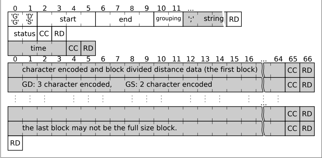
Figure 3.2 : GD, GS Message Format
