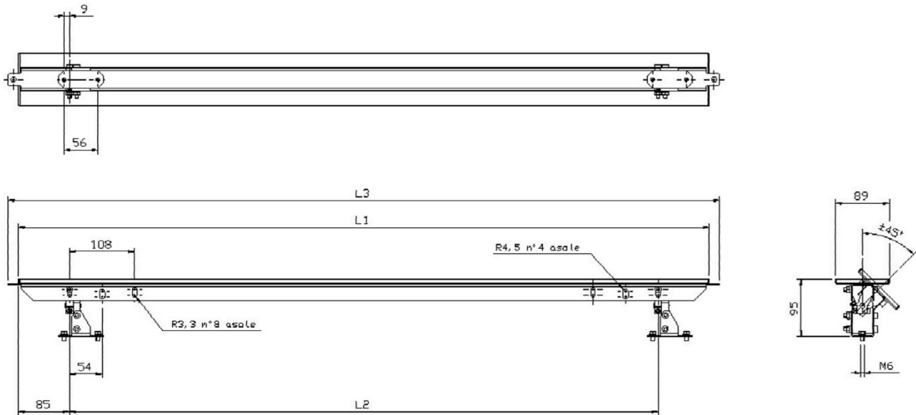
Fig 94 - Dimensions ( mm)
