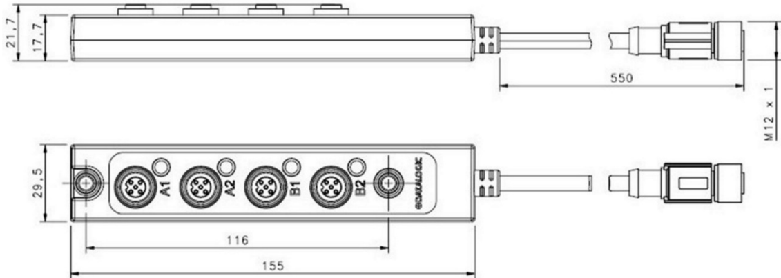
Fig 122 - Dimensions
