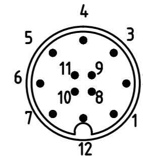
Ansicht auf Steckerkontakte
