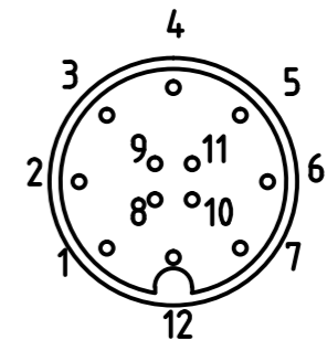
Ansicht auf Buchsenkontakte
