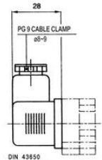
DIN 43950 IP65-ISO4400
