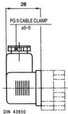
DIN 43950 IP65-ISO4400
