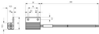
Termostat KTO 011 (NC)
