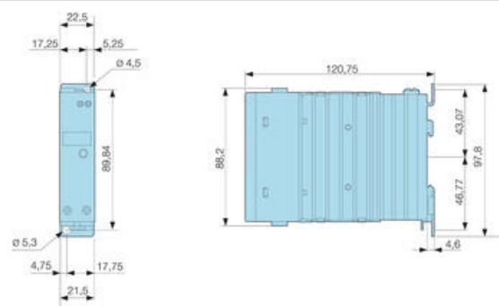
Prevedenie "relé"
