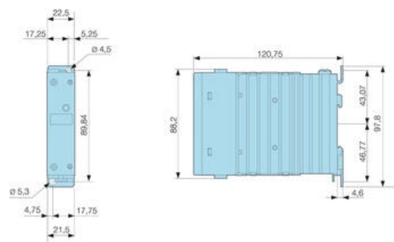
Prevedenie "stýkač"
