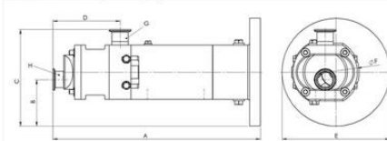
Mäz HYGHSPIN Extended kompaktmonterad (mm)
