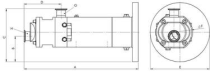
Mått HYDRISPIN Extended kompaktkonstrad (mm)
