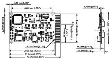
Figure 7.1. ISCM4805 / ISCM8005 dimensions
