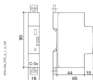
DIRIS Digiware C-31
