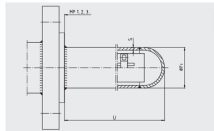
■ Thermowell (option)
